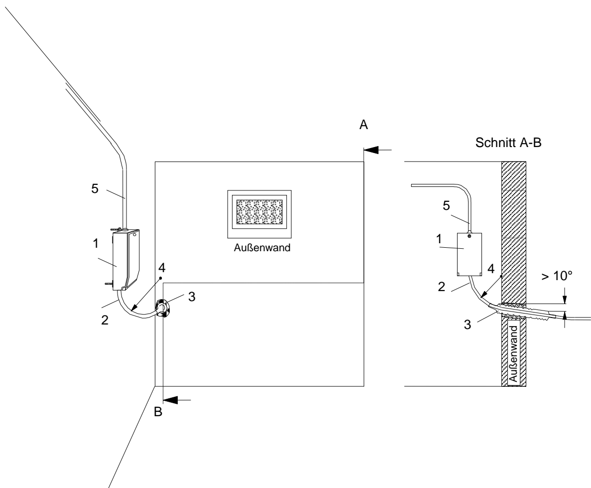
Abb. 6: Beispiel für einen Kabel-Netzanschluss, Innenanschlusstechnik
