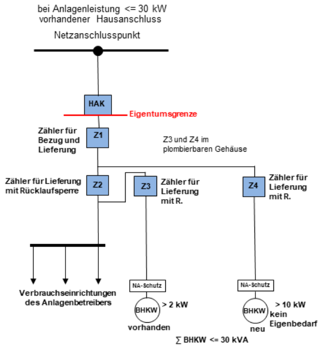
Abb. 14: Erzeugungsanlagen-Schaltungen E12
