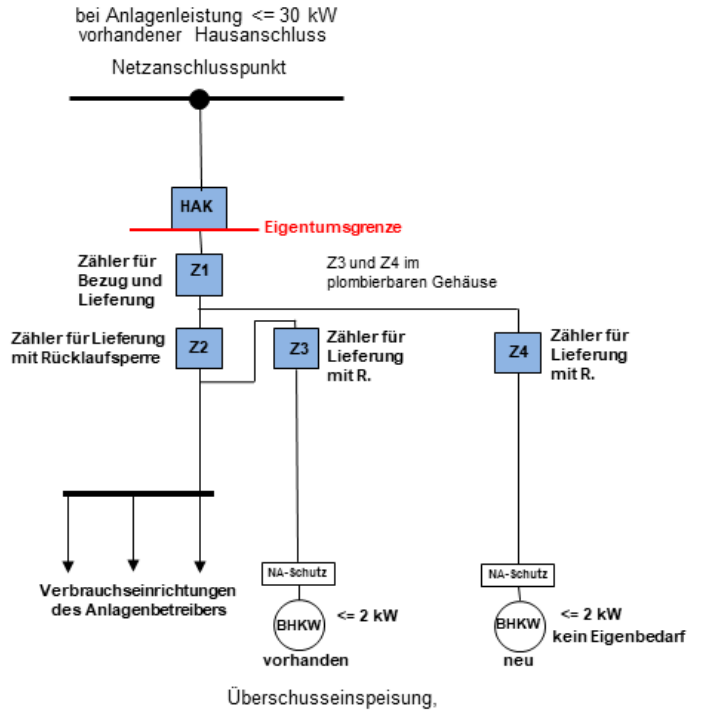
Abb. 13: Erzeugungsanlagen-Schaltungen E11
