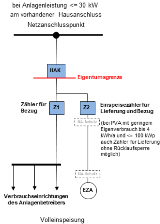
Abb. 3: Erzeugungsanlagen-Schaltungen E1
