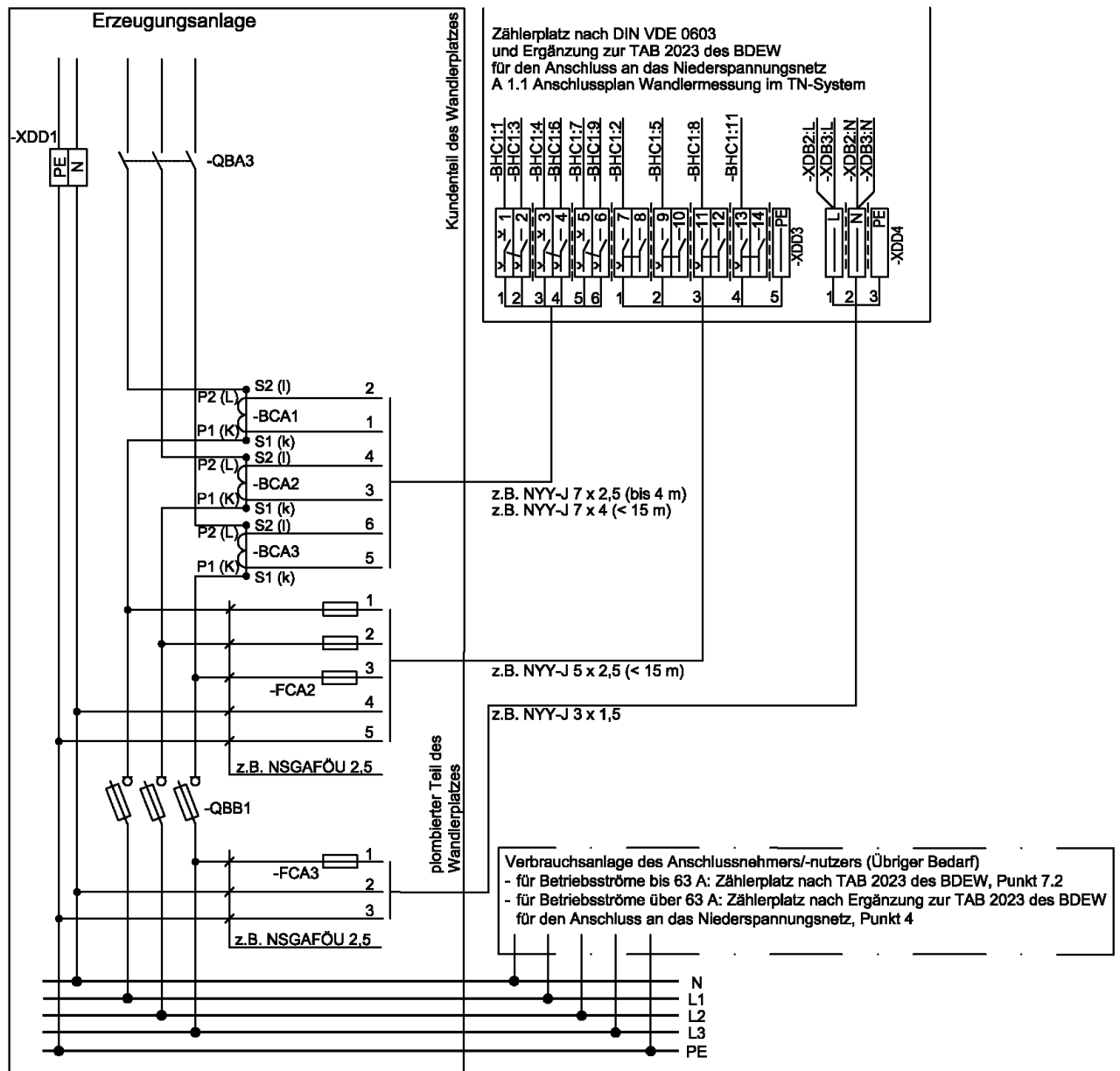
Abb. 19: Anlage mit Eigenerzeugung, Volleinspeisung über Wandlerzählung
