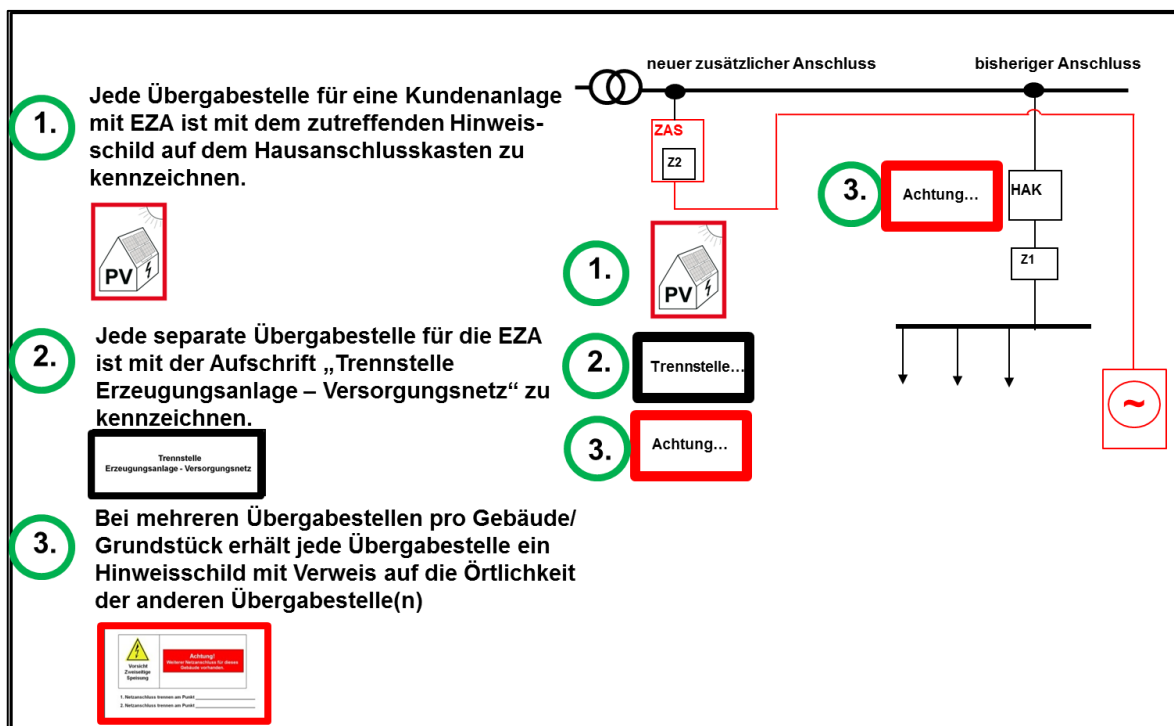
Abb. 14: Kennzeichnung der Kundenanlage mit Hinweisschildern „Erzeugungsanlage, Trennstelle und Übergabestelle“ (beispielhaft)
