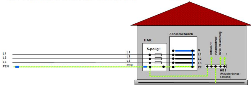
Abb. 19: Anschlussvariante bei MITNETZ STROM zur Innenanschlusstechnik (beispielhafte Darstellung)
