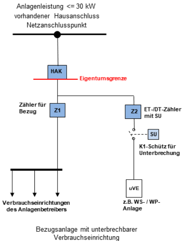
Abb. 2: Bezugsanlagen-Schaltungen B2
