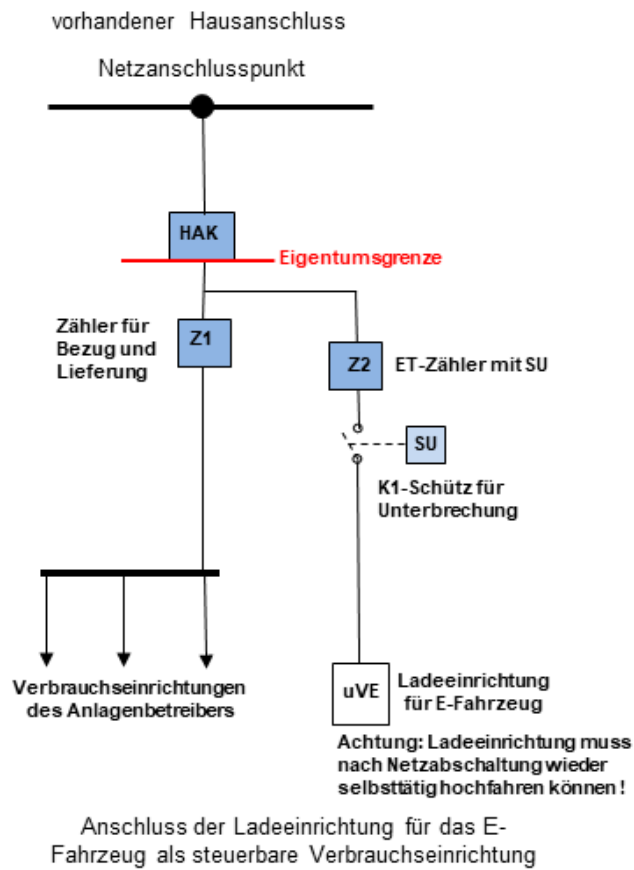
Abb. 37: Elektromobilität-Schaltungen EMob 2
