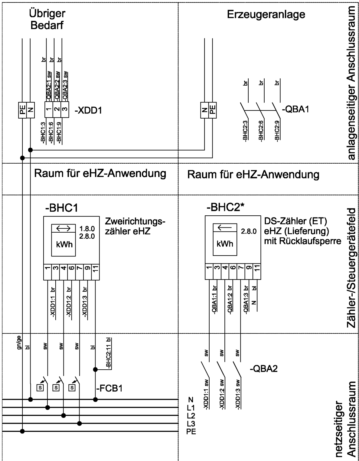
Abb. 24: Zählerschrank (BKE-I und zweifeldrigen Schrank)
