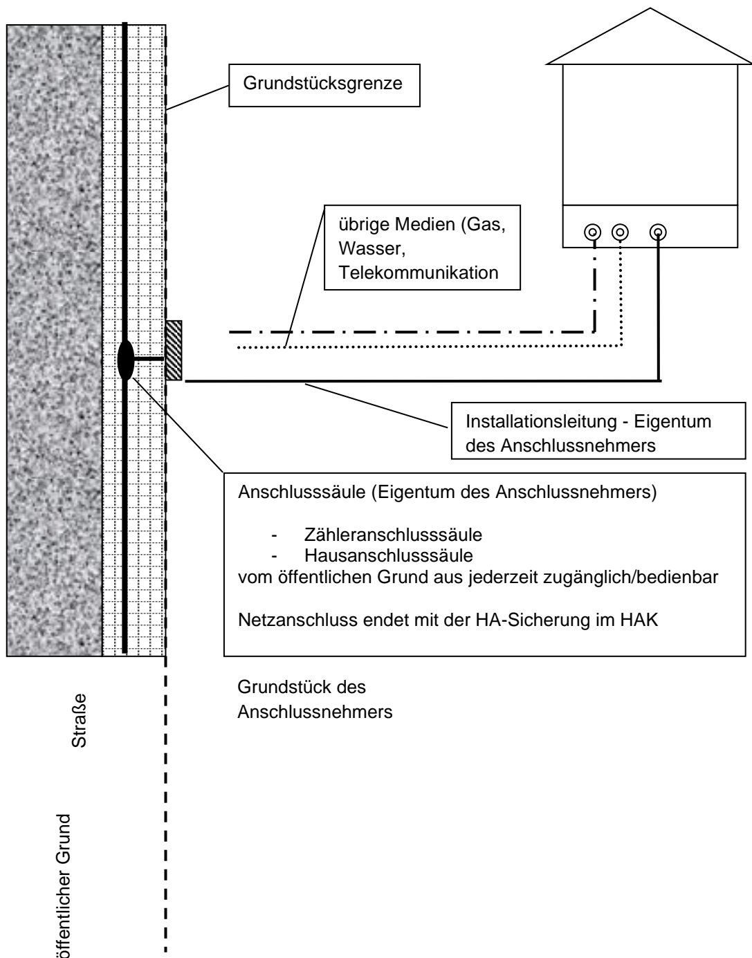
Abb. 5: Beispiel für Außenanschlusstechnik mit Anschlussssäule
