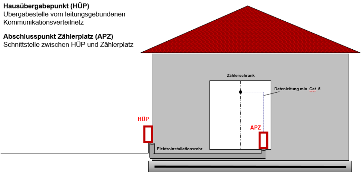
Abb. 8: Anbindung von Kommunikationseinrichtungen (beispielhaft)
